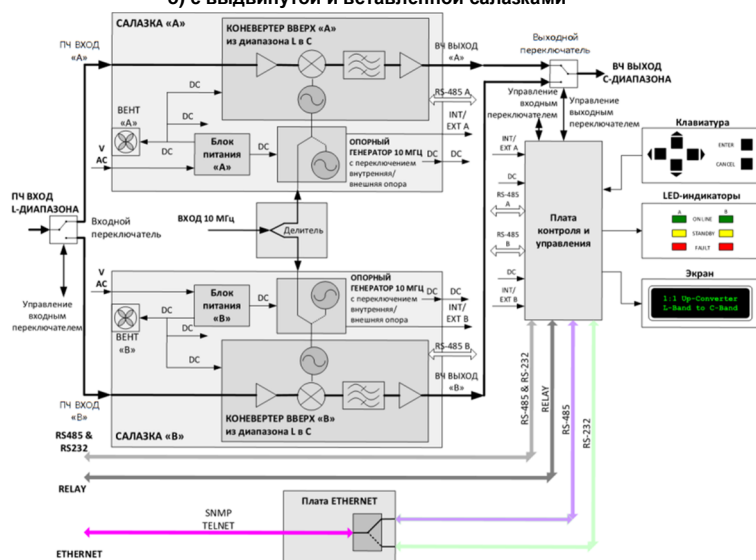
Рис.2: Структурная схема конвертера 1:1 из диапазона L в С
