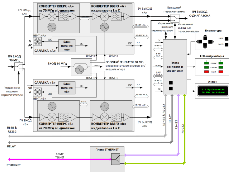
Рис.2: Структурная схема конвертера 1:1 из 70 МГц в С-диапазон
