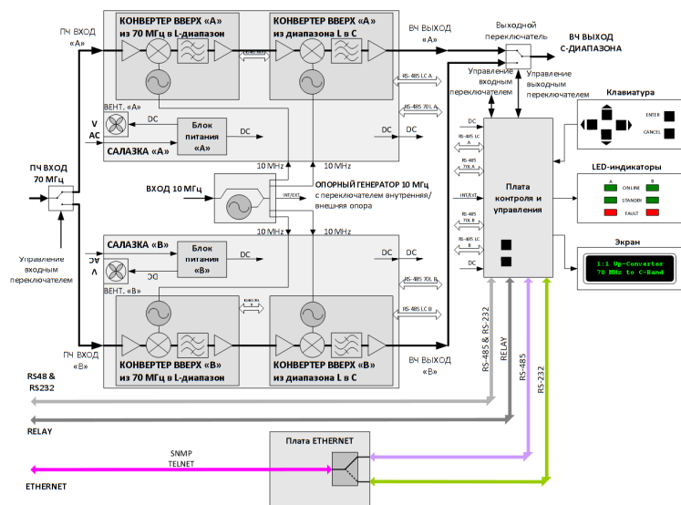
Рис.2: Структурная схема конвертера 1:1 из 70 МГц в С-диапазон
