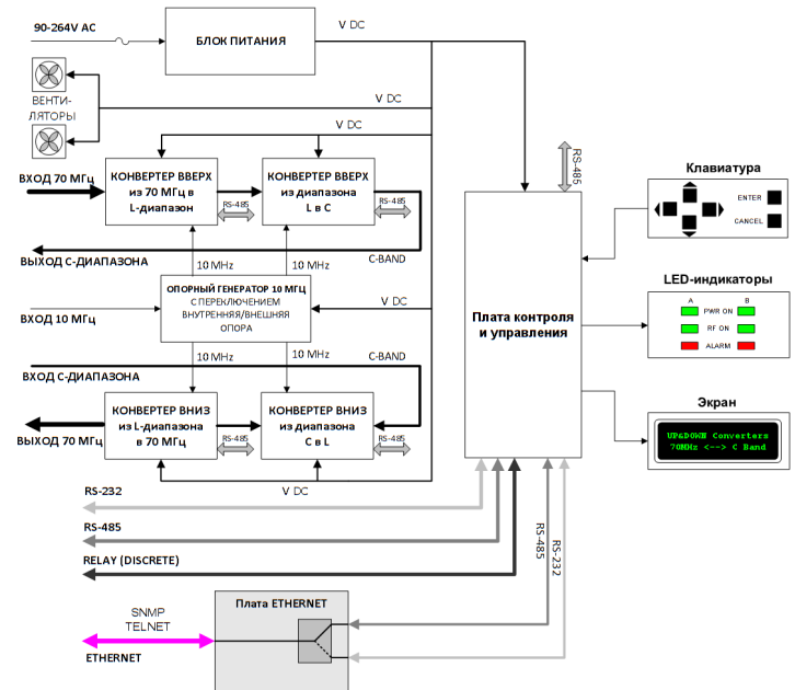
Рис.1: Структурная схема преобразователя вверх-вниз 70 МГц - С-диапазон
