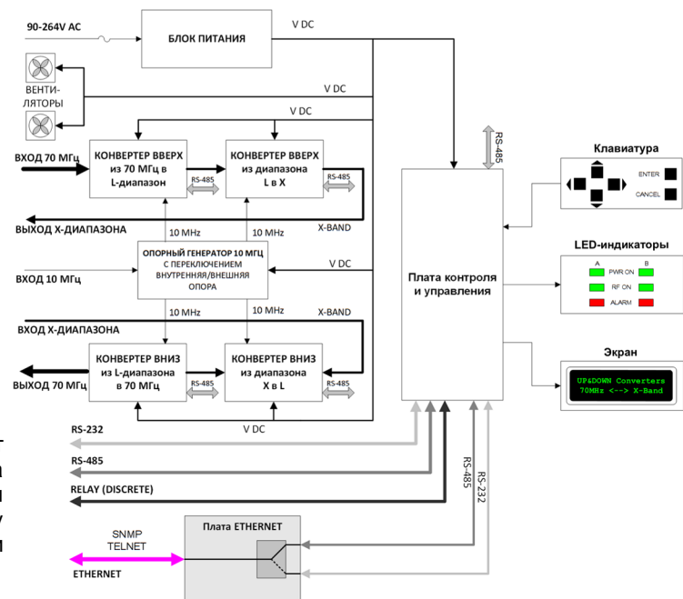
Рис.1: Структурная схема преобразователя вверх-вниз 70 МГц - X-диапазон
