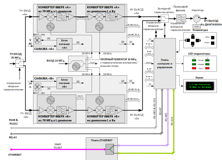
Рис.2: Структурная схема конвертера 1:1 из 70 МГц в Ku-диапазон
