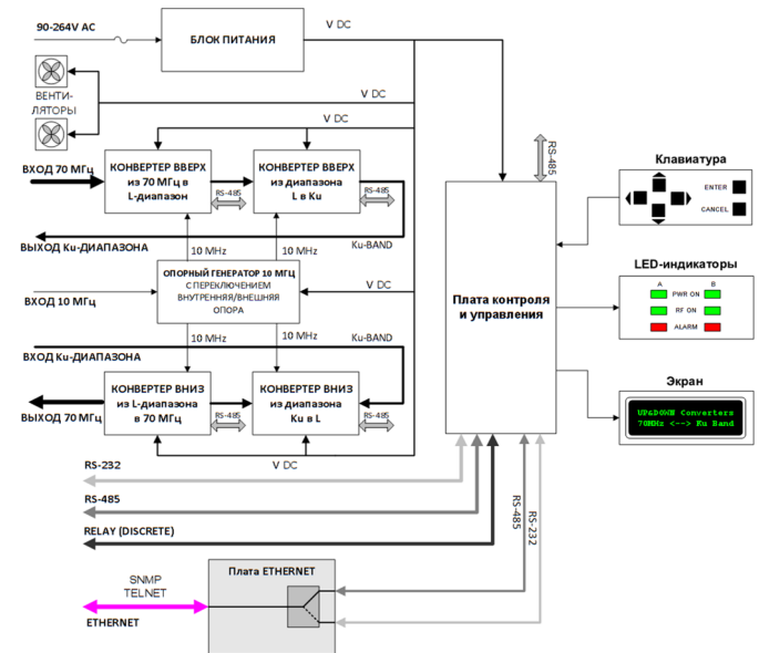
Рис.1: Структурная схема преобразователя вверх-вниз 70 МГц - Ku-диапазон
